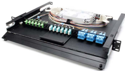
Distribuidor Optronics 1 UR
